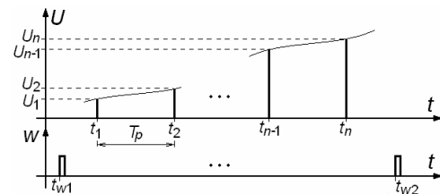
Rys. 1. Przebiegi czasowe sygnałów w przetworniku
