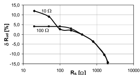
Rys. 8. Wpływ wartości rezystancji sond pomiarowych na wyniki pomiaru rezystancji udarowej uziemienia Fig. 8. Influence of value of the resistance of measurement probes on the results of measuring grounding impulse resistance
