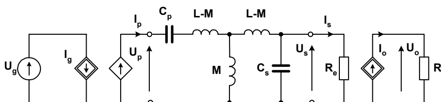
Ryc. 2. Model obwodowy systemu CEETS w analizie FMA
