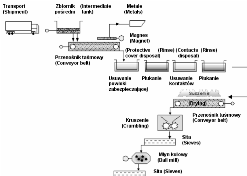
Rys. 7. Linia technologiczna do odzysku krzemu wysokiej czystości
