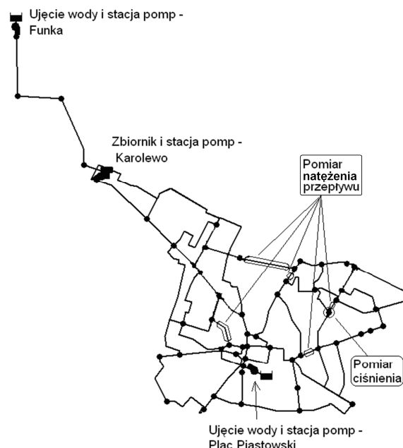
Rys. 4. Alokaacja pomiarów w sieci dla najlepszego punktu ze zbioru Pareto Fig. 4. The final hydraulic sensor placement in the network for the best point of Pareto set
