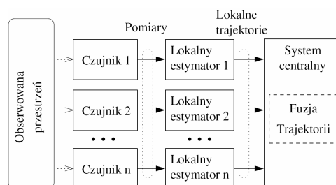
Rys. 1. Rozproszony system wyznaczania trajektorii Fig. 1. Distributed tracking system
