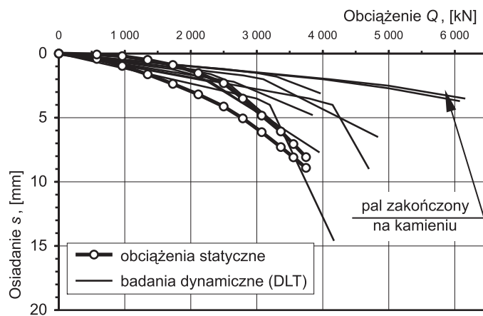
Rys. 6. Krzywe obciążenie-osiedlenie. Wiadukty nad ul. Puławską w Piasecznie
