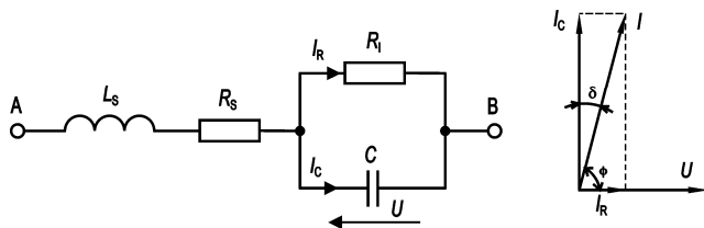
Rys. 2. Schemat zastępczy kondensatora o pojemności C , rezystancji upływności R_l , rezystancji szeregowej R_S i indukcyjności pasożytniczej L_S z wykresem wskazującym zależność fazowych między napięciem na kondensatorze U oraz jego prądem I_c ; I_r – prąd płynący przez rezystancję R_l
