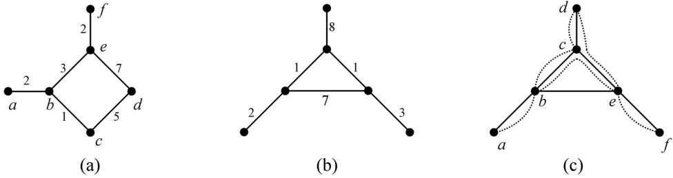
Rys. 1. Przykładowe umieszczenie (c) ważonego grafu (a) w grafie (b)
