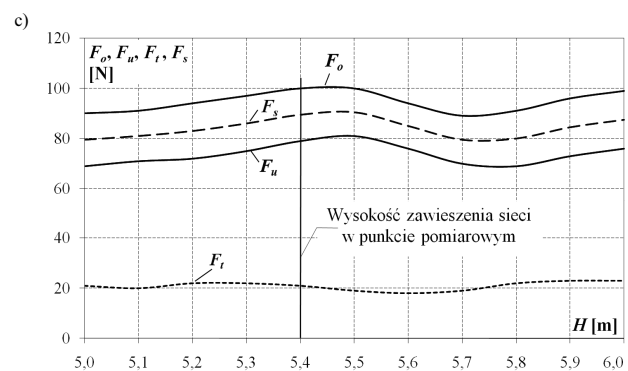
Rys. 7. Charakterystyki współpracy odbieraka z siecią: a) charakterystyki uniesienia przewodu jezdnych w zależności od siły statycznej odbieraka i prędkości pojazdu; b) przebieg uniesienia przewodu dla wybranego odbieraka; c) charakterystyka statyczna sił nacisku przy obniżaniu F_o i unoszeniu F_u odbieraka, wartości siły średniej F_s oraz podwójnej siły tarcia F_t – dla odbieraka z rys. b
