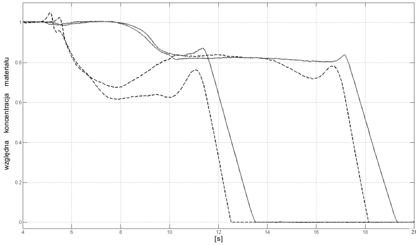
Rys. 7. Zmiany koncentracji piasku zagęszczonego dla pikselu zlokalizowanego: przy ścianie (p(1, 15)) – linia ciągła; w środku przekroju poprzecznego (p(15, 15)) – linia przerywana (krótsze charakterystyki przedstawiają zmiany koncentracji dla wysokości h = 1,5\text{m} , dłuższe dla h = 1,0\text{ m} ) (ściana szorstka)
