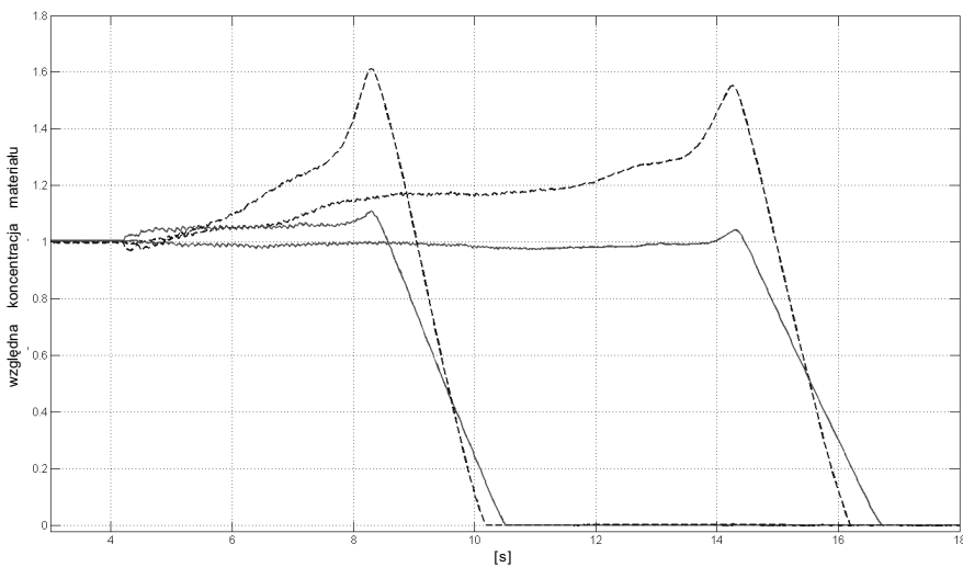
Rys. 1. Zmiany koncentracji piasku luźnego w przypadku ściany gładkiej dla piksela zlokalizowanego: przy ścianie ( p(1, 15) ) – linia ciągła; w środku przekroju poprzecznego ( p(15, 15) ) – linia przerywana (krótsze charakterystyki przedstawiają zmiany koncentracji dla wysokości h = 1,5 m, dłuższe dla h = 1,0 m)
