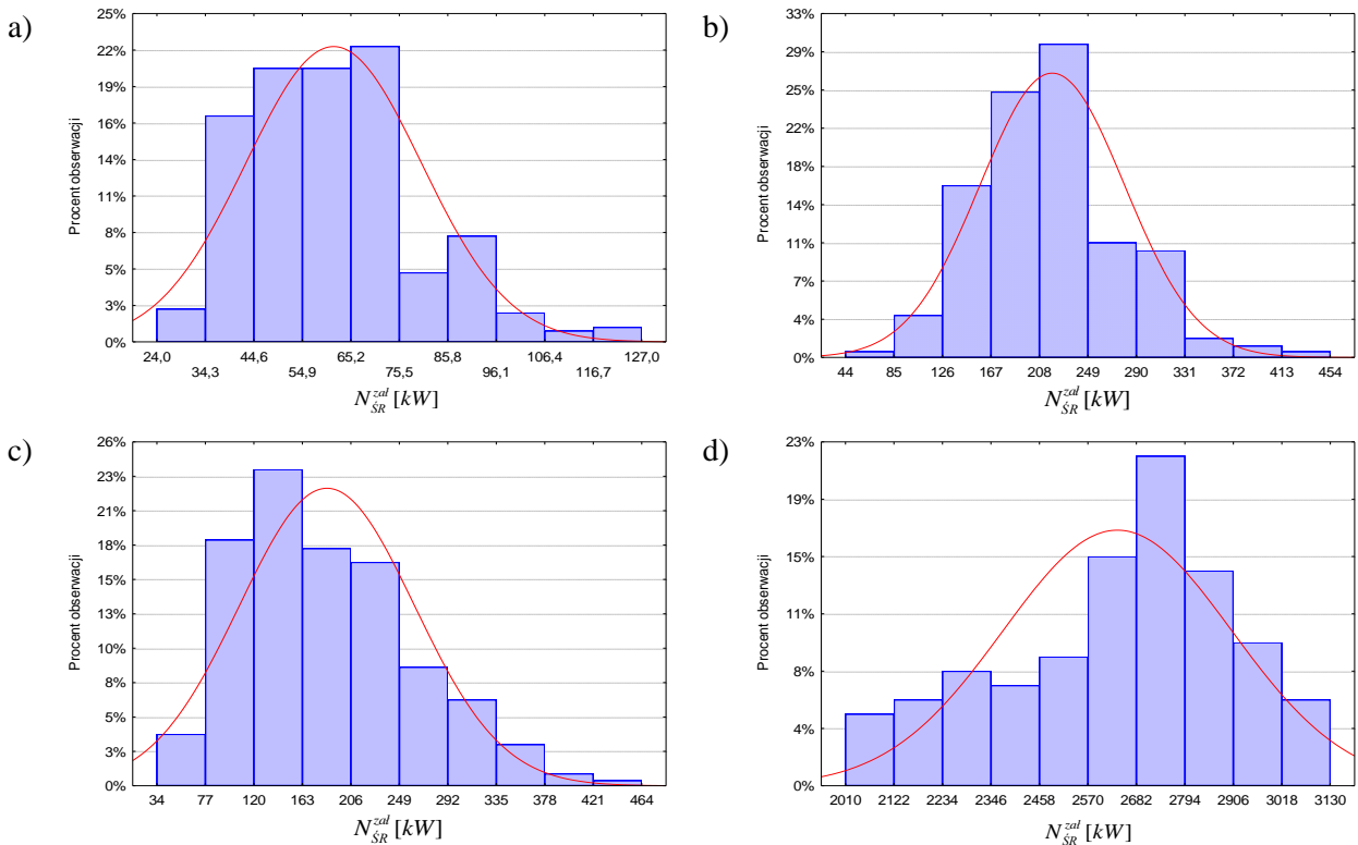
Rys. 2. Histogramy obciążeń śrub napędowych pogłębiarek ssących nasiębiernych podczas prac związanych z załadunkiem: a) „Kostera”, b) „Bukowski”, c) „Łęgowski”, d) „Geopotes 15” Fig. 2. Load distributions of propellers of trailing suction hopper dredger during dredging: a) “Kostera”, b) “Bukowski”, c) “Łęgowski”, d) “Geopotes 15”
