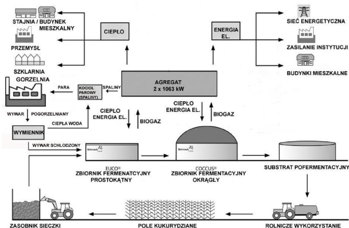
Rys. 3. Schemat instalacji wytwarzania i utylizacji biogazu w Gorzelnii Liszkowo [7] Fig. 3. Schema of biogas generation and utilisation system in Liszkowo Distillery [7]
