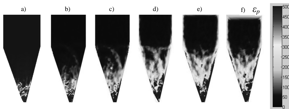
Rys. 2. Zmiana odkształceń postaciowych \varepsilon_p w zagęszczonym piasku średnioziarnistym d_{50} = 0,8 mm w silosie ze ścianami gładkimi i przepływem masowym: a) 1 s, b) 2 s, c) 3 s, d) 5 s, e) 7 s, f) 8 s (wypływ grawitacyjny)
