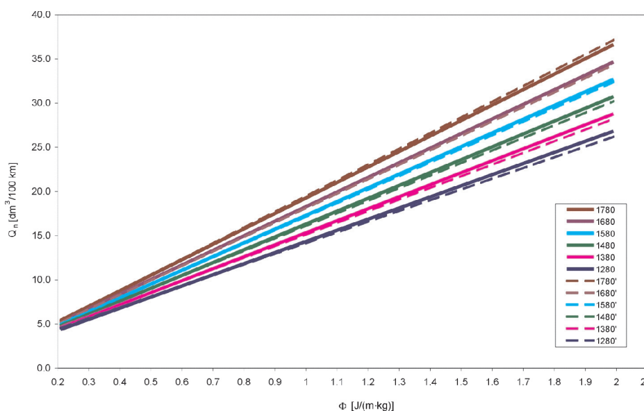
Fig. 14. Characteristic family (9) created for the vehicle 3 Rys. 14. Rodzina charakterystyk (9) utworzonych dla pojazdu 3
