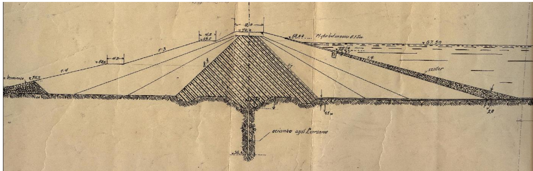
Rys. 1. Przekrój poprzeczny zapory [3]
