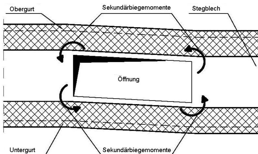
Bild 3: Sekundärbiegemomente infolge Querkraftbeanspruchung
