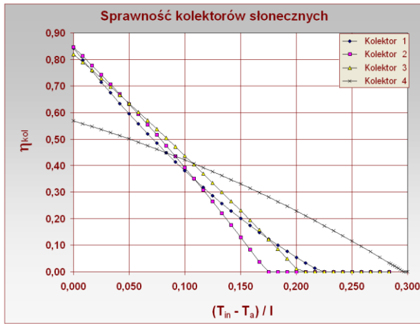
Rys. 1. Graficzna ilustracja zależności (1) opisujących sprawność kolektorów słonecznych
