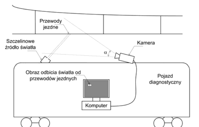
Rys. 1. Koncepcja bezkontaktowego pomiaru położenia przewodu jezdnej sieci trakcyjnej
