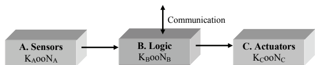
Fig. 1. Architecture of E/E/PES or SIS for realization of safety-related functions Rys. 1. Architektura systemu E/E/PE lub SID do realizacji funkcji związanych z bezpieczeństwem
