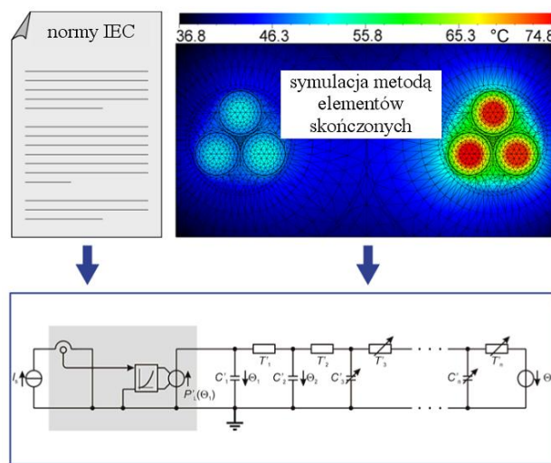
Rys. 4. Model RTTR dla kabli wysokonapięciowych tworzony na podstawie danych pomiarowych temperatury ekranu lub poprzez analizę w programie polowym
