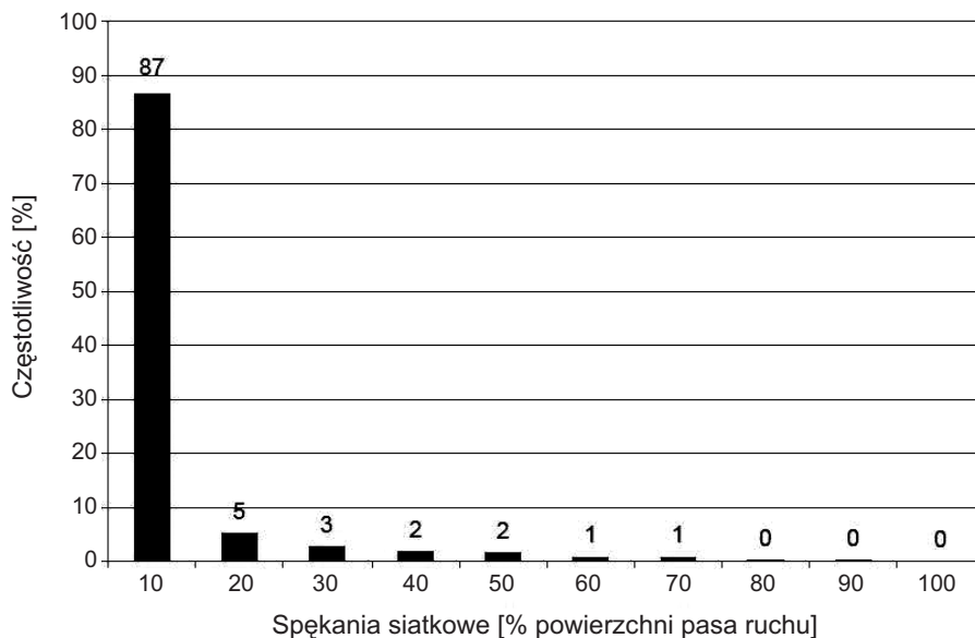
Rys. 8. Częstotliwość występowania spękań o różnej intensywności na odcinkach doświadczalnych nawierzchni LTPP
