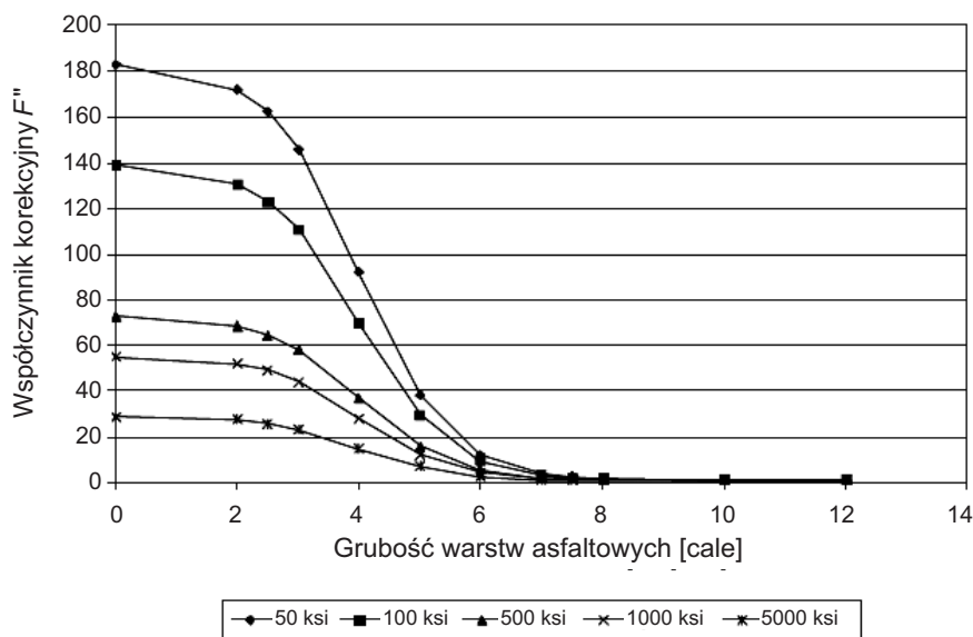
Rys. 1. Funkcja sigmodalna F'' przy różnych sztywnościach warstwy Fig. 1. Sigmoidal function F'' for different layer stiffness
