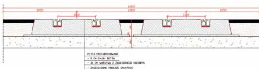
4. Przekrój poprzeczny pasa autobusowo-tramwajowego w Toruniu
