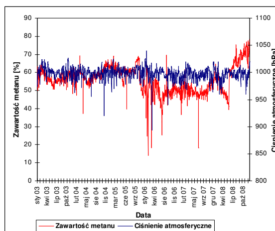
Rys. 7. Zależność zmian zawartości metanu od ciśnienia atmosferycznego (lata 2003÷2008)
