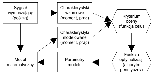
Rys. 1. Optymalizacja z wykorzystaniem algorytmu genetycznego
