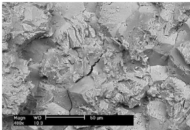
Rys. 17. Pęknięcie zimne w złączu implant. Przełom kruchy transkryształiczny i częściowo międzykryształiczny. W centralnej części zdjęcia widoczne międzykryształiczne pęknięcia prostopadłe do powierzchni przełomu [43]
