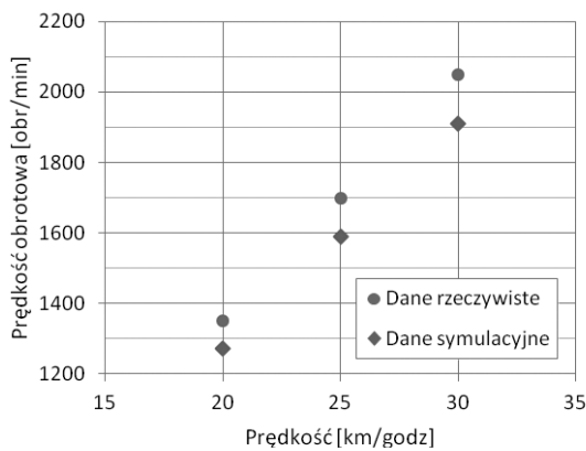
Rys. 9. Prędkość obrotowa pojazdu – bieg 2
