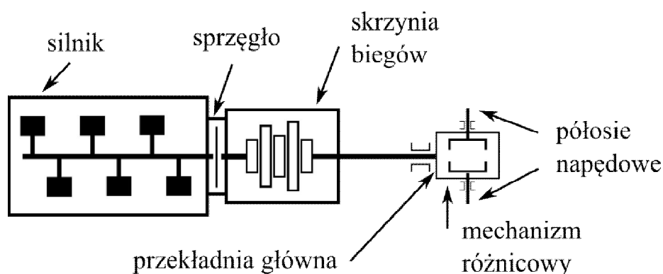
Rys. 1. Schemat ideowy układu napędowego
