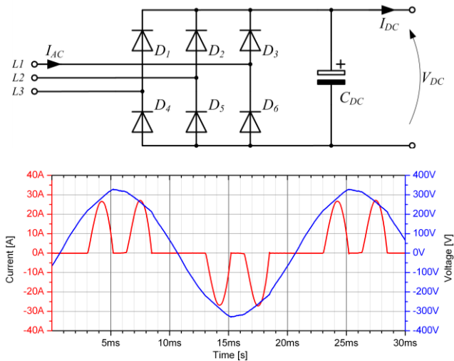
Rys. 2. Klasyczny trójfazowy 6 pulsowy prostownik diodowy oraz typowo odkształcony przebieg prądu wejściowego pobieranego z sieci zasilającej
