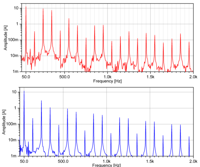
Rys. 5. Porównanie widm składowych harmoniczných prądu wejściowego prostownika 6 pulsowego z obciążeniem pojemnościowym: bez filtracji (wykres górny) oraz z filtracją pasywną (wykres dolny)
