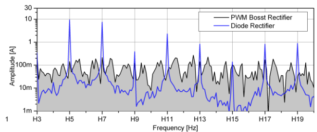
Rys. 8. Porównanie widm zaburzeń przewodzonych małej częstotliwości prądu wejściowego przekształtnika diodowego oraz tranzystorowego
