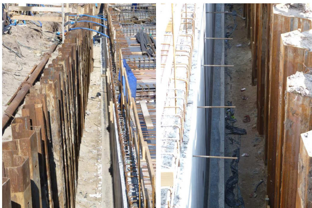
Rys. 4 – Obudowa wykopu
