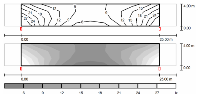
Rys. 7. Rozkład natężenia oświetlenia na drodze rowerowej; lampy diodowa – izolinie
