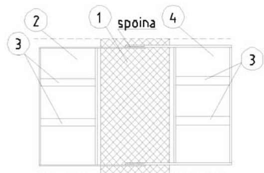
Rys. 4. Widok z góry na skrzynię zamontowane na stanowisku badawczym: 1 – żelbetonowa kładka; 2 – skrzynia z podklejoną do dna izolacją; 3 – usztywnienia łebkowe; 4 – skrzynia bez izolacji
