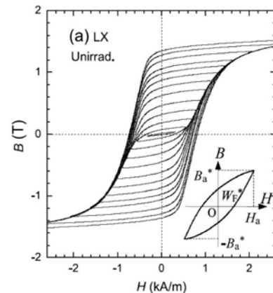
Rys. 4. Kolejne pętle histerezy zmierzone w metodzie A1 oraz parametry tych pętli Fig. 4. Following hysteresis loops measured in the A1 method and parameters of the loops
