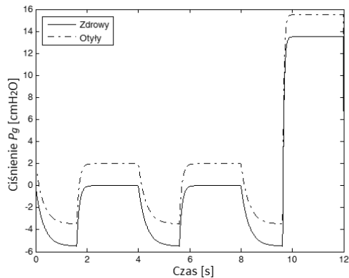
Rys. 2. Przebieg ciśnienia wywieranego przez ruchy przepony [2, 8] Fig. 2. Time course of pressure caused by diaphragm [2, 8]
