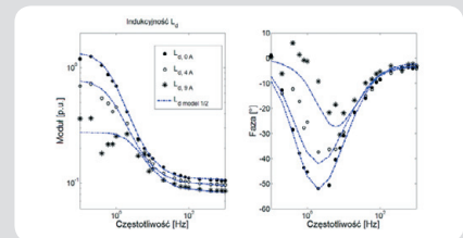
Rys. 11. Porównanie charakterystyk indukcyjności operatorowej L_{1d} maszyny synchronicznej z wynikami pomiarów częstotliwościowych SSFR w warunkach nasycenia
