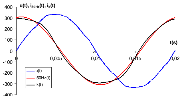
Rys. 8. Porównanie skorygowanego przebiegu prądu upływowego i_k(t) z prądem harmonicznej podstawowej 50 Hz i_{50Hz}(t) wynikającej z analizy algorytmem FFT przebiegu rzeczywistego i(t)
