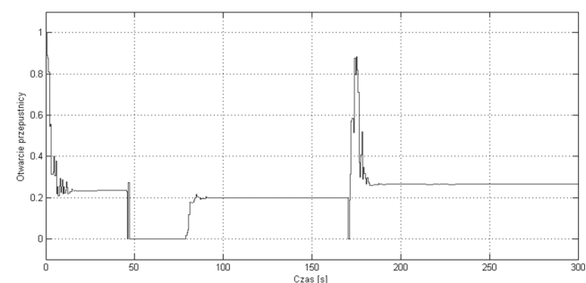
Rys. 6. Układ regulacji MPC – bieg 3, brak zakłóceń Fig. 6. MPC control system – gear 3, without disturbances
