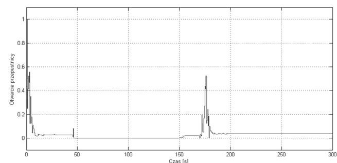
Rys. 5. Układ regulacji MPC – bieg 1, brak zakłóceń Fig. 5. MPC control system – gear 1, without disturbances
