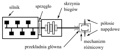
Rys. 1. Schemat ideowy układu napędowego samochodu Fig. 1. Schematic diagram of the car propulsion system
