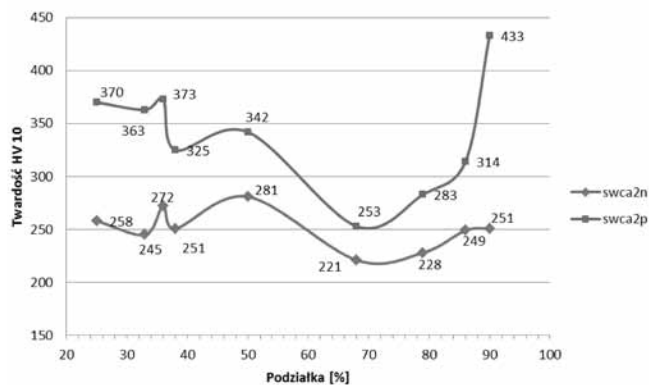
Rys. 14. Rozkład twardości stref swca2n i swca2p w pierwszej napoinie na stali S355J2G3 w zależności od podziałki ściegów
