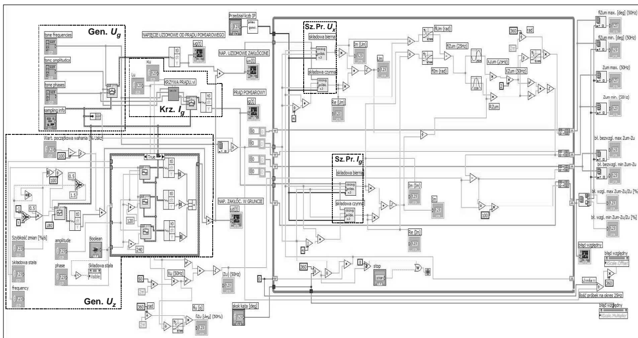
Rys.3. Diagram aplikacji
