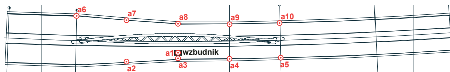
Rys. 13. Rozmieszczenie punktów pomiarowych podczas badań z użyciem wzbudnika elektrodynamicznego
