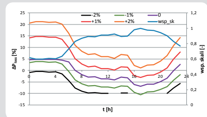
Rys. 4. Procentowa różnica strat w sieci bez i z optymalizacją
