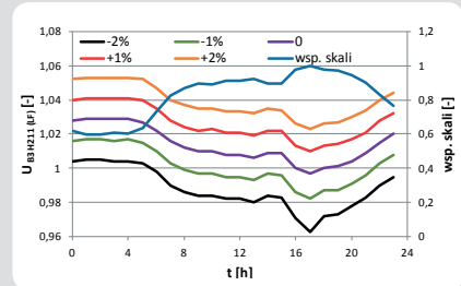
Rys. 5. Napięcia w wybranym węźle sieci: B3H211, bez optymalizacji (LF)
