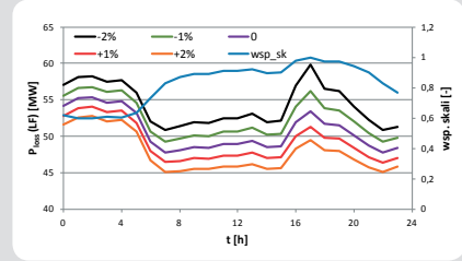
Rys. 2. Straty mocy w sieci. Wpływ zmiany napięć zadanych generatorów. Bez optymalizacji (LF)
