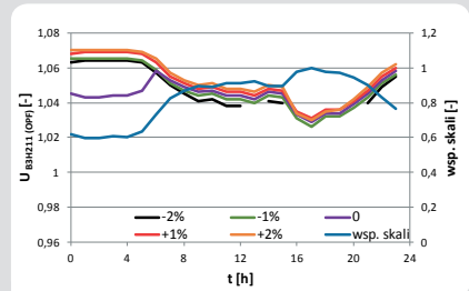
Rys. 6. Napięcia w wybranym węźle sieci: B3H211, z optymalizacją (OPF)
