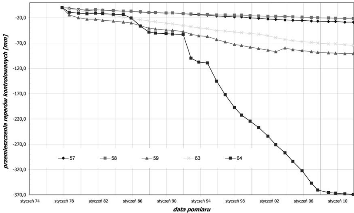
Rys. 7. Osiedlenia reperów na zaporce ziemnej Smukała (w rejonie dawnej elektrowni)
