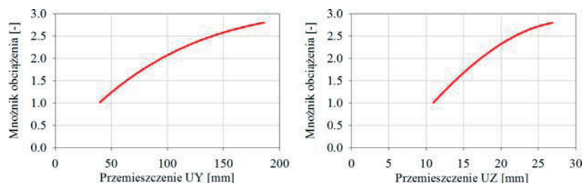
Rys. 7. Przeszczenia poziome UY (prostopadle do estakady) i pionowe UZ punktu na pasie górnym dźwigara 11-12 w środku rozpiętości
