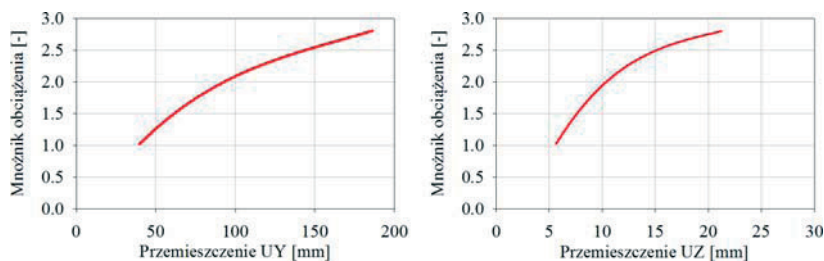
Rys. 6. Przeszczenia poziome UY i pionowe UZ punktu na szczycie słupa 11
