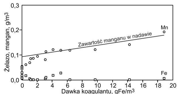
Rys. 2. Zawartość związków żelaza i manganu w permeacie podczas oczyszczania wody podziemnej w zintegrowanym procesie koagulacja/mikrofiltracja Fig. 2. Iron and manganese content in permeate upon groundwater treatment in integrated coagulation/microfiltration process
