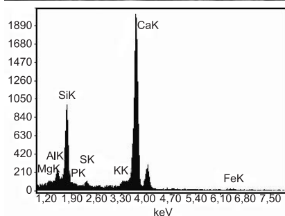
Fot. 4. Widok ogólny i skład pierwiastkowy (SEM/EDS) mikrostruktury betonu z udziałem mikrosfer w spoiwie, po 360 dniach przechowywania w środowisku wody (aut. E. Haustein)
