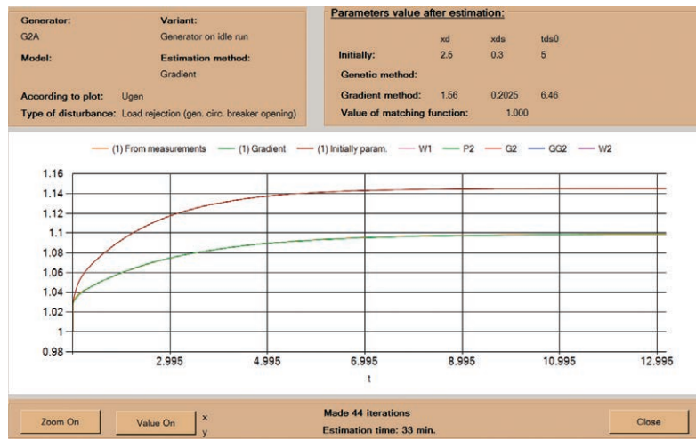
Rys. 1. Wyniki estymacji parametrów w osi d dla modelu hydrogeneratorsza (krok 2)
