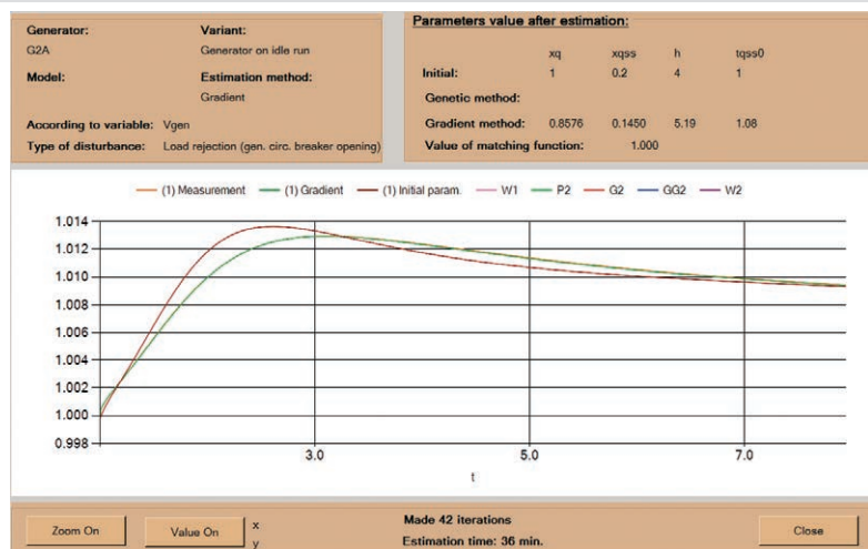
Rys. 2. Wyniki estymacji parametrów w osi q dla modelu hydrogeneratorsza (krok 3)
