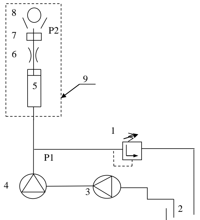
Rys. 3. Schemat hydrauliczny zestawu nagniatającego: 1- zawór przelewowy, 2- zbiornik z płynem chłodząco-smarującym, 3- pomocnicza pompa zasilająca agregat, 4- pompa wysoko-ciśnieniowa, 5- siłownik w narzędziu, 6- dławik, 7- czujnik siły, 8- gniazdo z kulką nagniatającą, 9- zespół narzędzia
