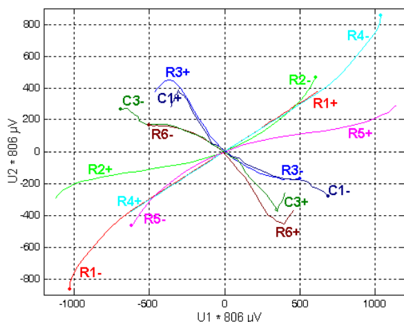
Rys. 7. Eksperymentalne krzywe lokalizacyjne dla układu badanego (rys. 2) na płaszczyźnie pomiarowej
