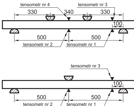
Rys. 10. Stanowiska dla zginania 4- oraz 3-punktowego
