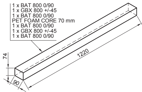
Rys. 9. Geometria belek
