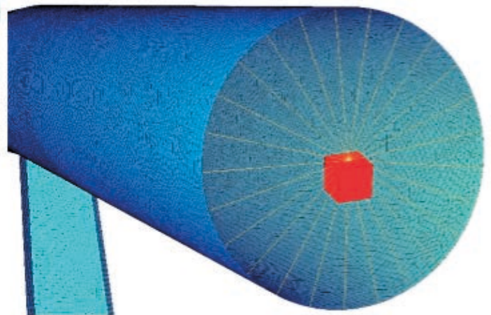
Rys. 7. Wizualizacja modelu obliczeniowego (W14) wersja pierwotna a) widok ogólny i szczegółowy modelu, b) sztywne elementy belkowe łączące krawędzie elementów powłokowych z punktem brzegowym
