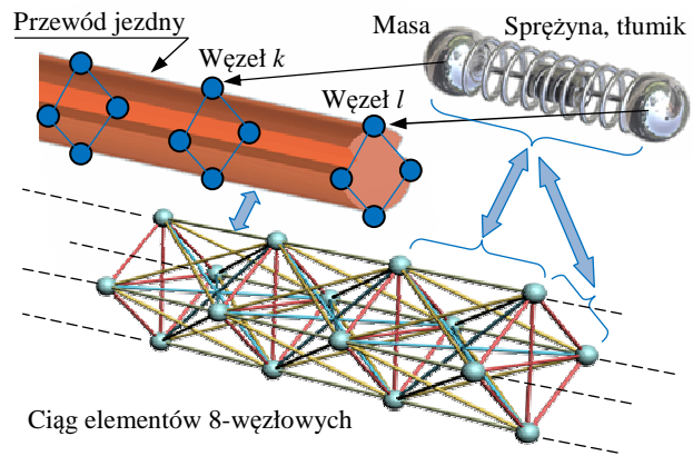
Rys. 3. Koncepcja podziału przewodu jezdny i podtrzymującego na zbiór skupionych elementów zachowawczych (masy, sprężyny) i elementów dysypatywnych (tłumiki)
